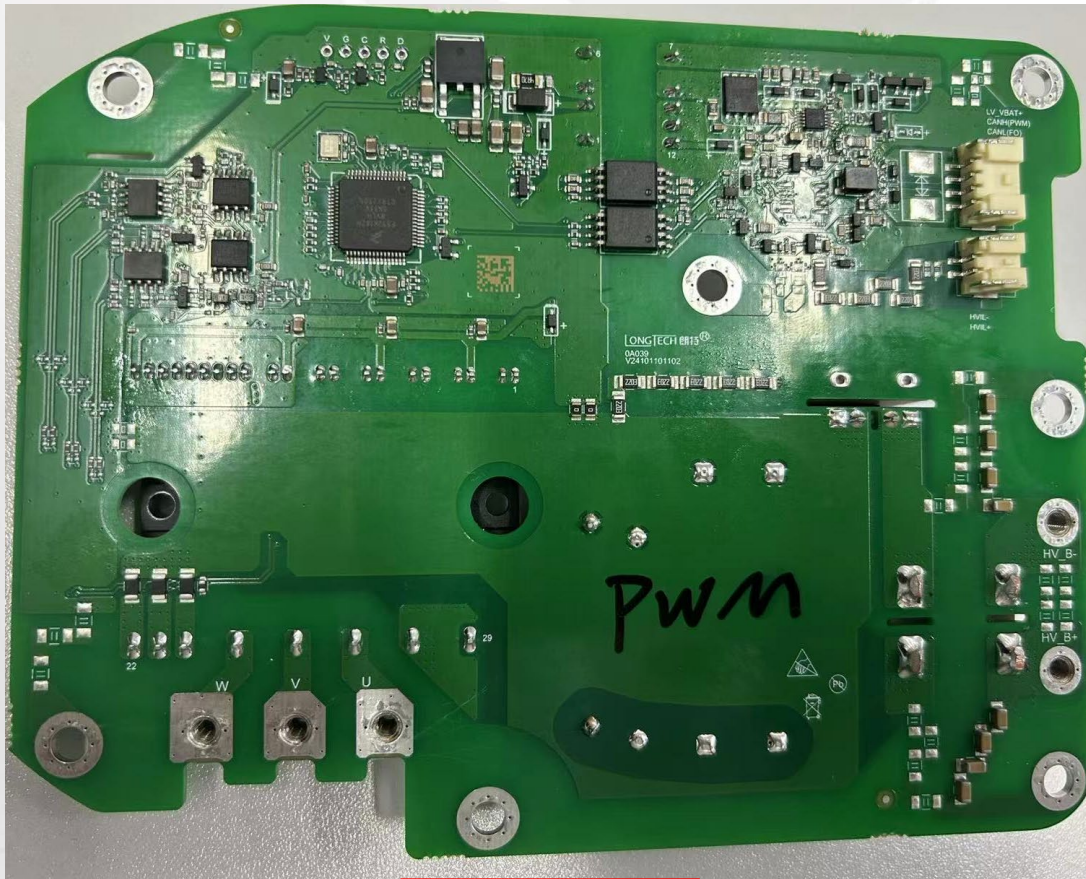
控制器正面
