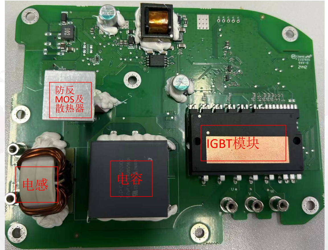
控制器反面
